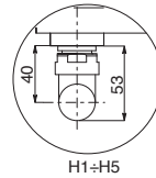
Maatvoeringen van de aansluitingen "Elegant" Cordivari
